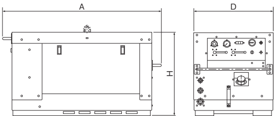
寸法表
