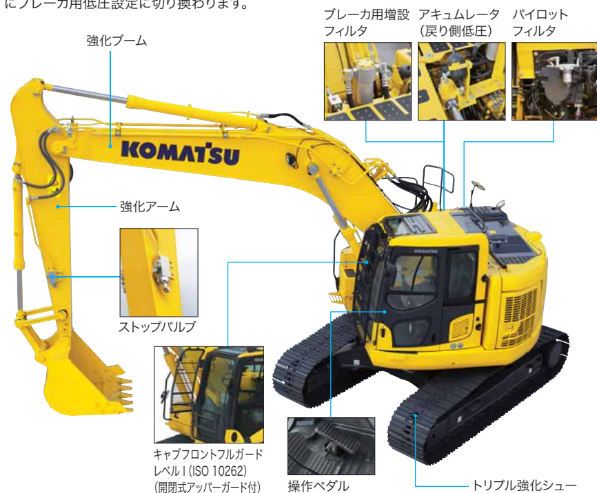
クラッシャなどのアタッチメント〈アタッチメントモード時〉
