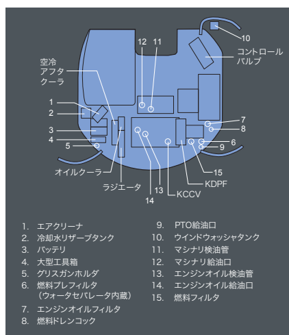
ウォーターセパレータ機能付 燃料プレフィルタ
